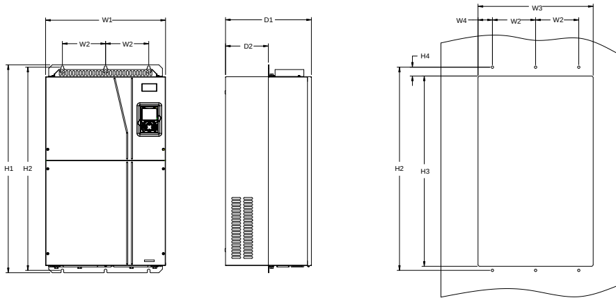
图 C.11 380V 132-200kW 法兰安装示意图
