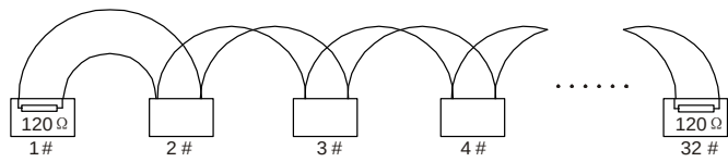
图 10.2 菊花接法现场接线图
