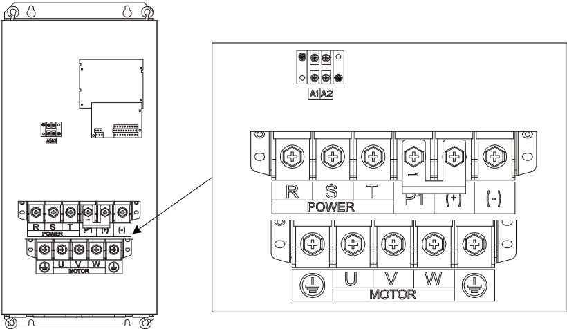
图 4.13 660V 55~132kW 主回路端子示意图
