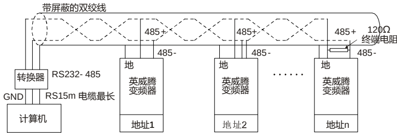
图 10.4 菊花接法运用图
