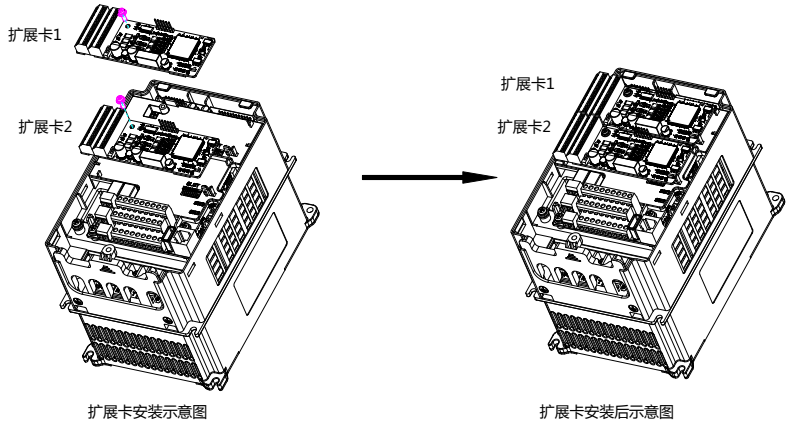
图 A.2 5.5KW（含）以下功率段效果图
