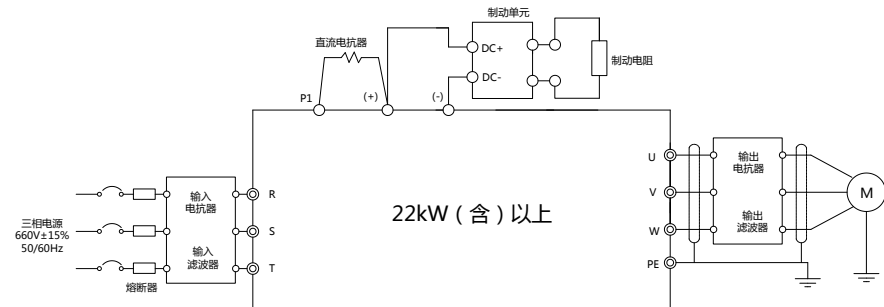
图 4.8 AC 3PH 520V(-15%)~690V(+10%)主回路接线图
