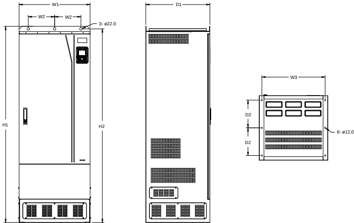
图 C.20 660V 400-630kW 落地安装示意图
