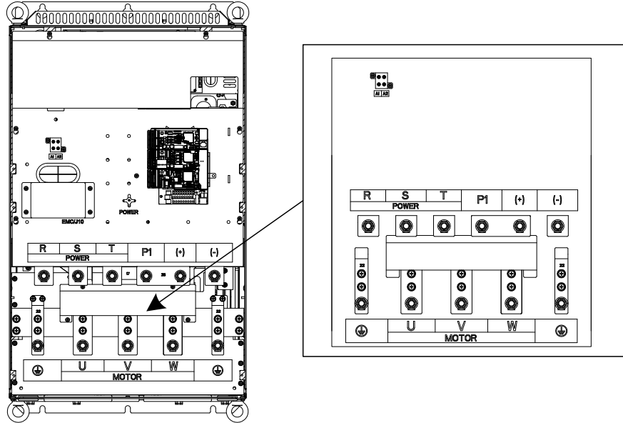
图 4.14 380V 132~200kW、660V 160~220kW 主回路端子示意图
