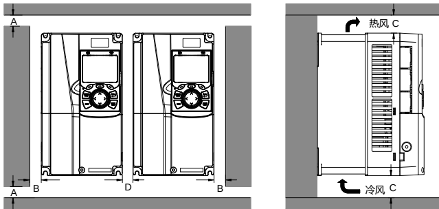
图 4.4 并行安装
