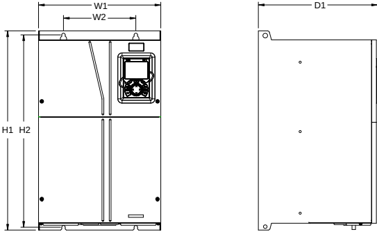
图 C.6 380V 90-110kW 壁挂安装示意图
