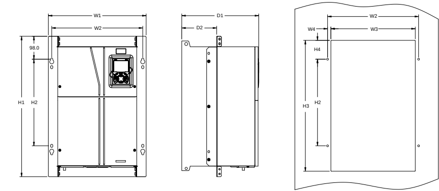
图 C.17 660V 22-132kW 法兰安装示意图
