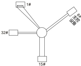
图 10.5 星形接法
