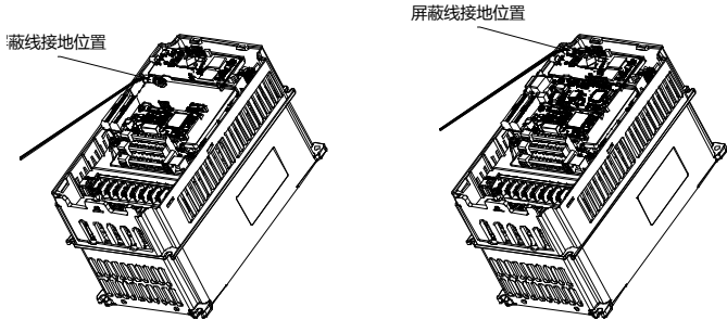
图 A.4 扩展卡地线连接示意图
