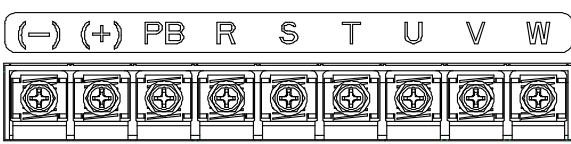
图 4.10 三相 380V 30-37kW 主回路端子示意图
