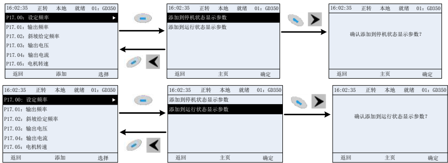
图 5.13 添加参数示意图 1
