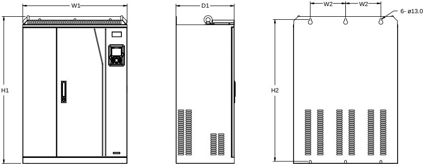
图 C.16 660V 250-355kW 壁挂安装示意图
