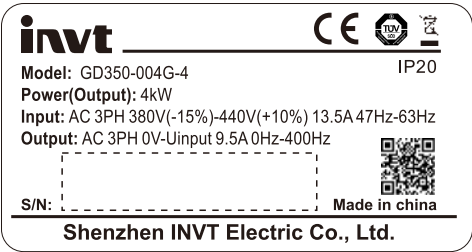
图 3.5 产品铭牌
