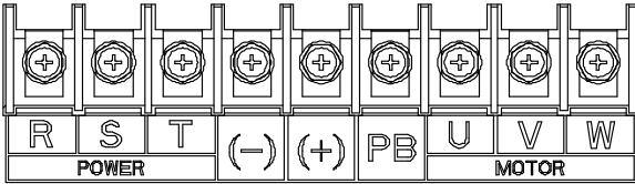
图 4.11 三相 380V 45-110kW 主回路端子示意图
