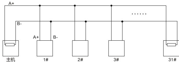
图 10.3 菊花简化接线图
