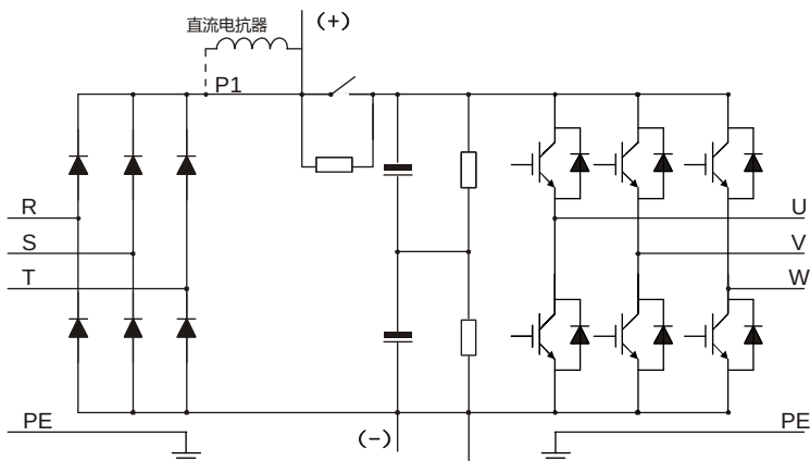
图 3.3 380V（大于 132kW（含））主回路简图
