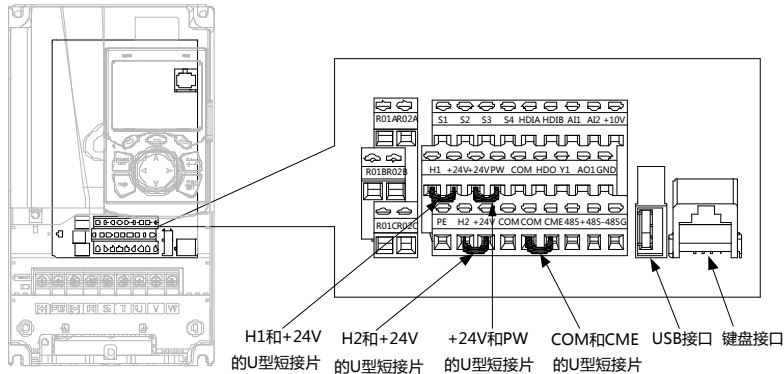
图 4.19 U 型短接位置示意图
