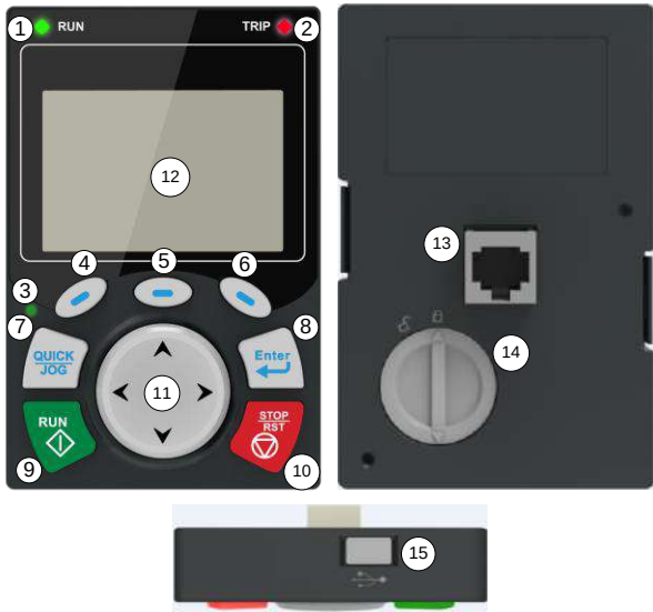
图 5.1 键盘示意图
