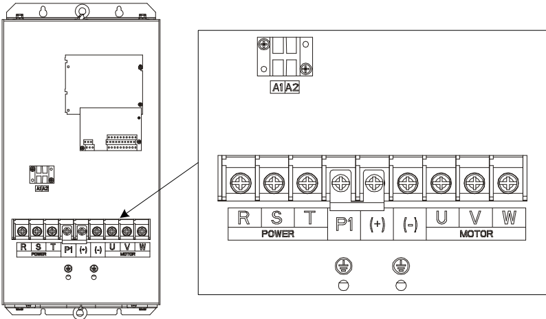
图 4.12 660V 22~45kW 主回路端子示意图
