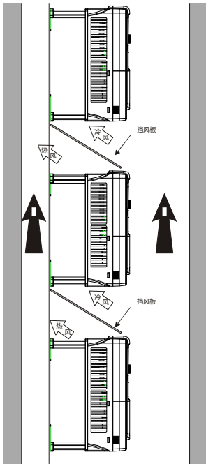
图 4.5 垂直安装
