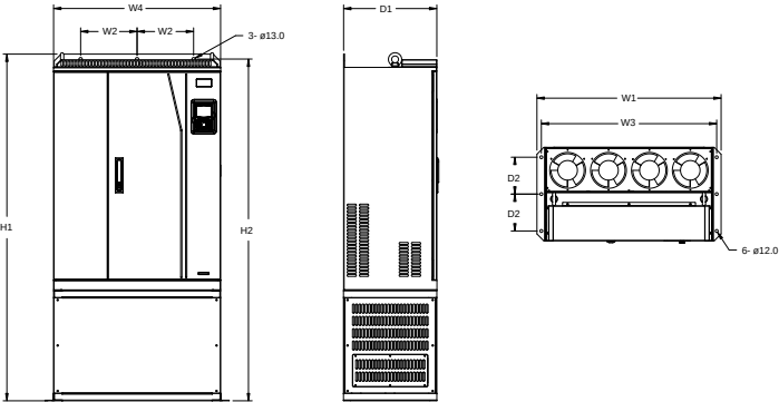
图 C.19 660V 250-355kW 落地安装示意图
