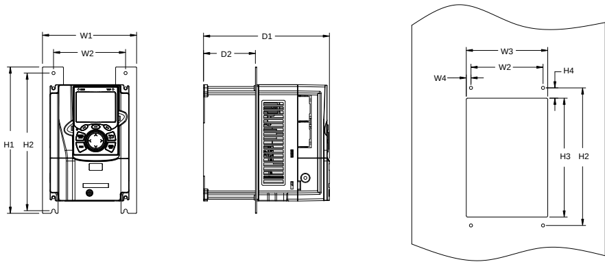
图 C.9 380V 1.5-75kW 法兰安装示意图
