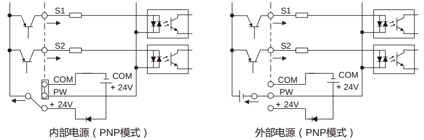
图 4.21 PNP 模式示意图
