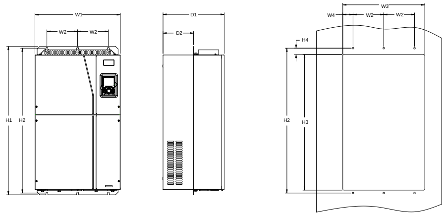
图 C.18 660V 160-220kW 法兰安装示意图表 C.5 660V 法兰安装尺寸表（单位：mm）
